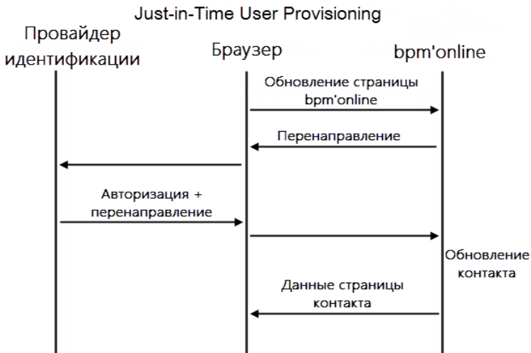
Рис. 461 — Схема обновления данных при использовании Just-in-Time User Provisioning
